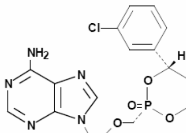
Pradefovir (INN) 17 .
