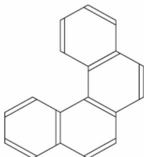
Naftalen
