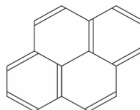
Kondensert kinolin
