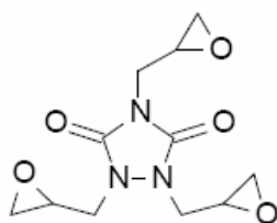
Anaxirone (INN)
